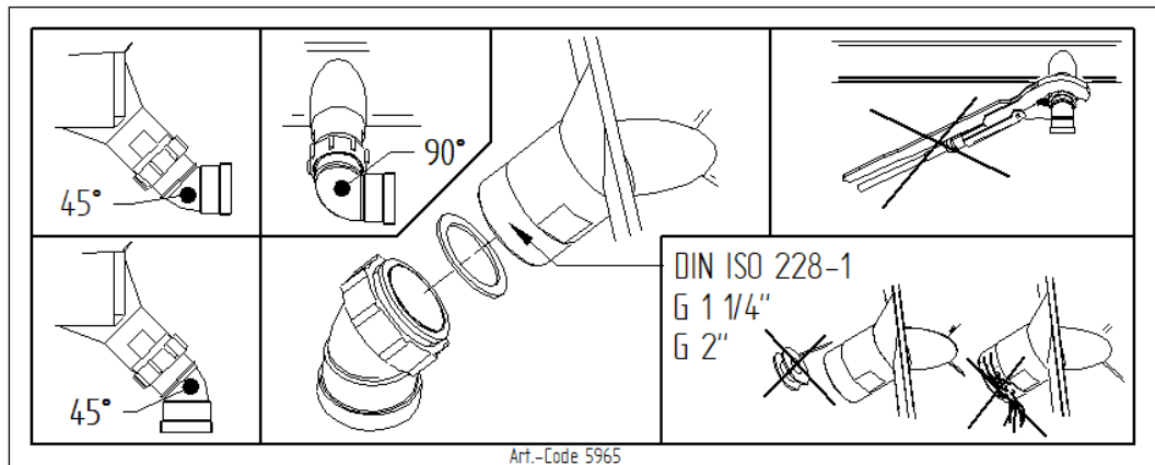
5965 - Warnhinweis Wannenablauf
